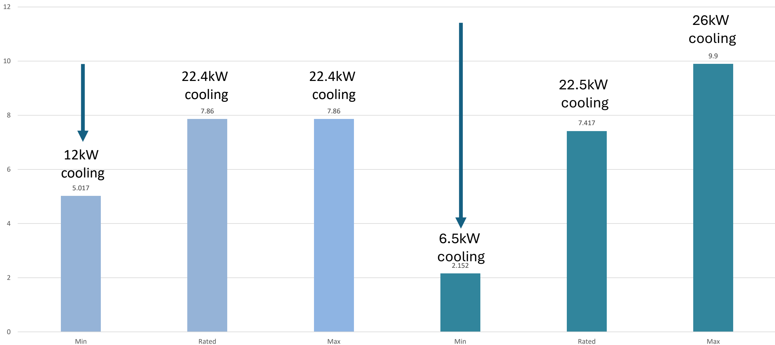
Power Input (kW)
